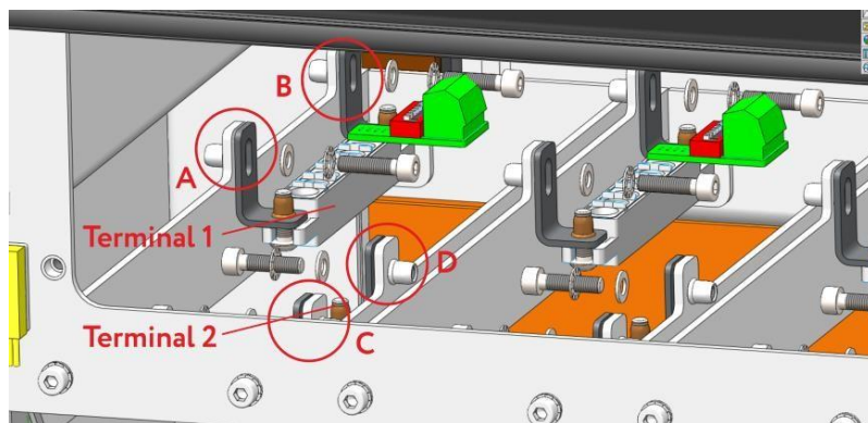
Рисунок 5.18. Подключение модулей
