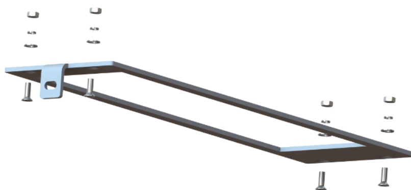
Рисунок 5.14. Кронштейн модуля
