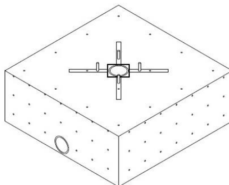
Рисунок 5.6. Трехмерная схема бетонного основания
