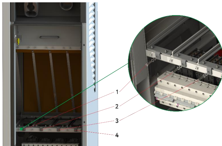
Рисунок 5.13. Место установки зарядных модулей
