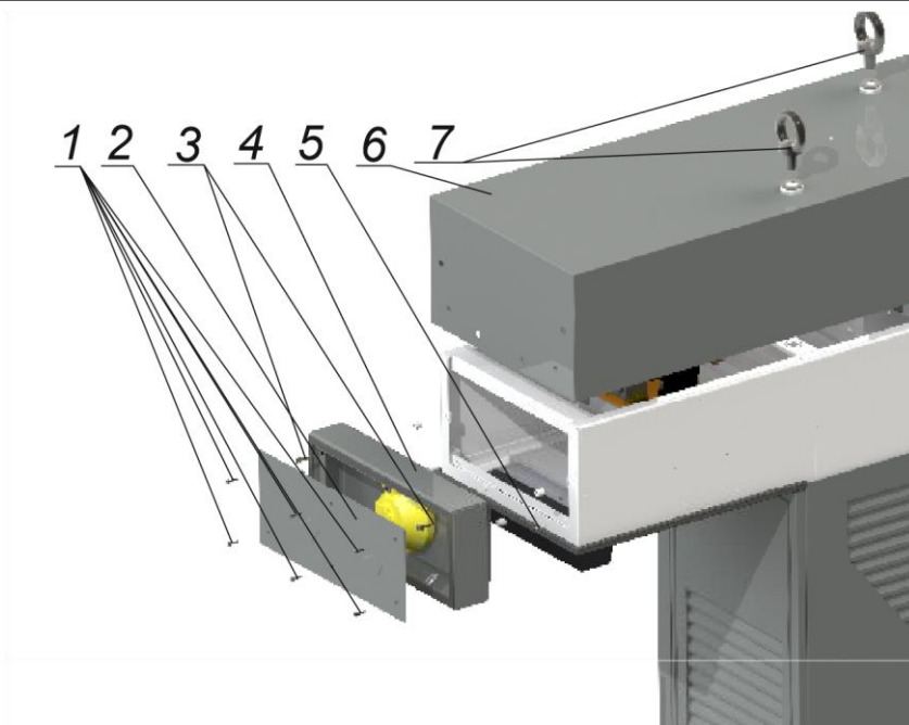
Рисунок 7.7. Расположение реле постоянного тока
