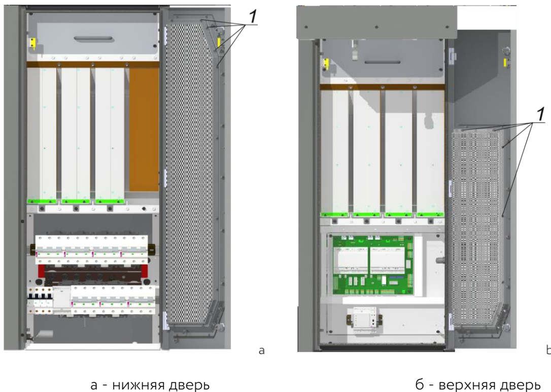
Рисунок 7.1 Расположение фильтров
