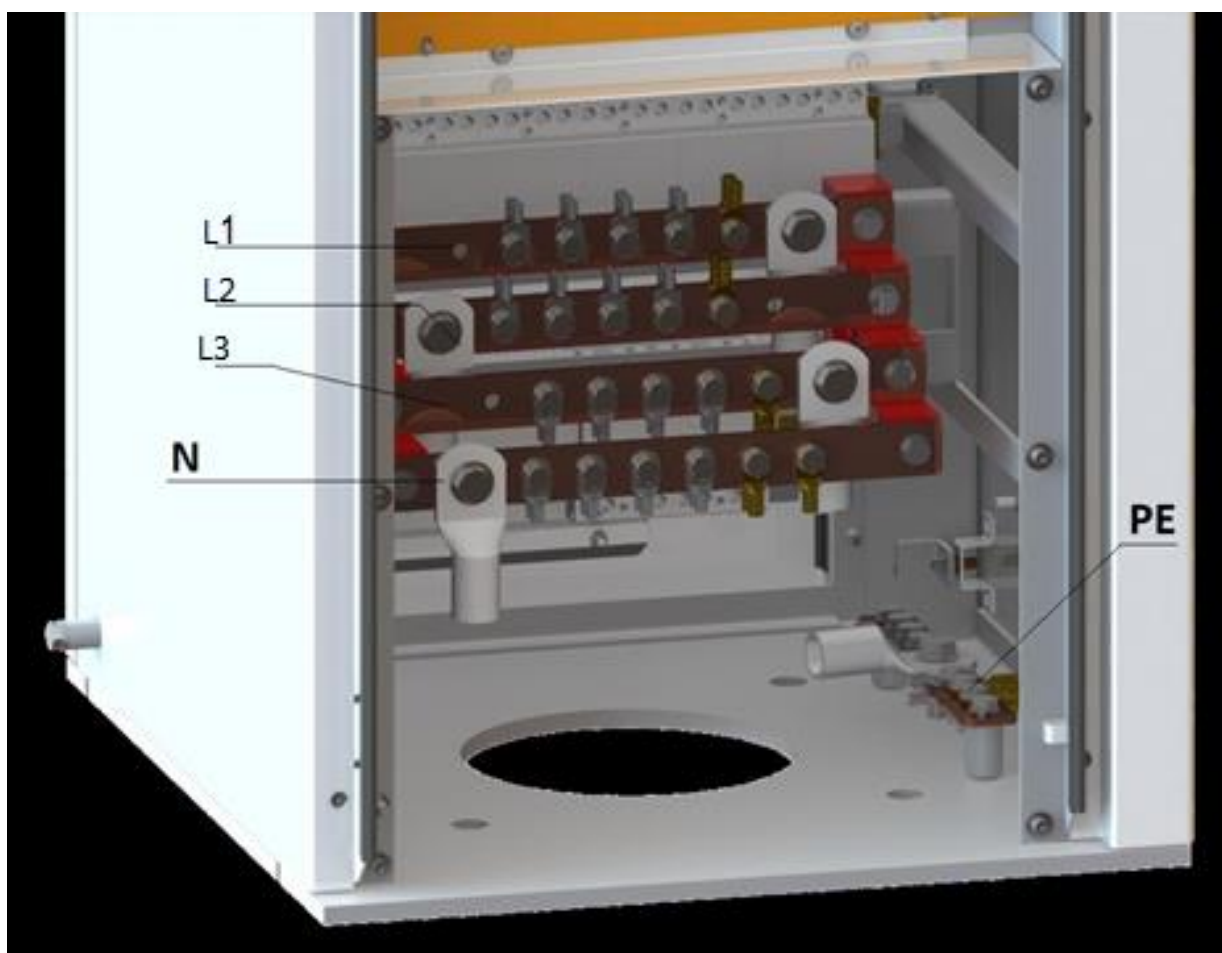
Рисунок 5.9. Входные шины
